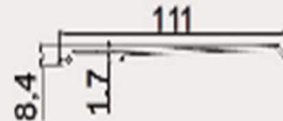
7 .PERFIL CIERRE FRONTAL
