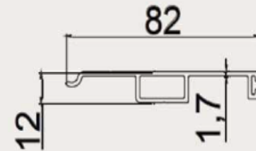
6 . PERFIL CIERRE LATERAL
