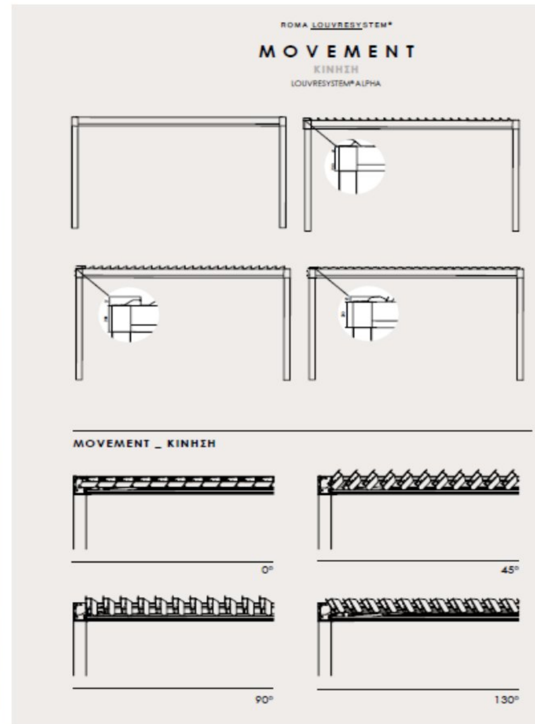
Detalle del movimiento de las lamas.
