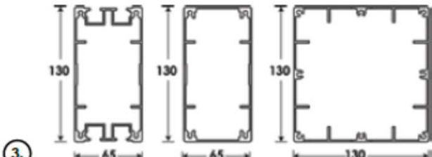
3. Columns
