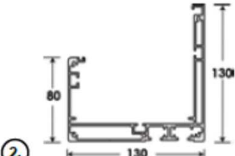
2. Rain Gutter
