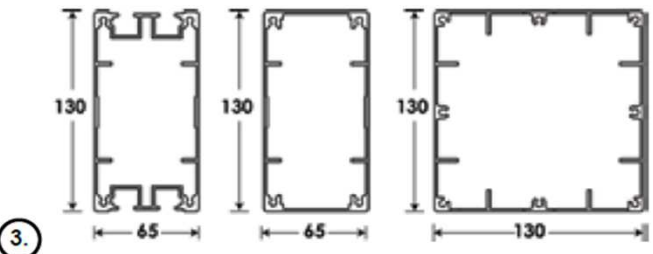
3. Columns
