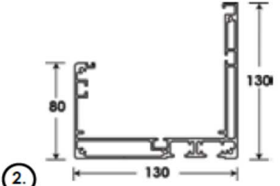
2. Rain Gutter
