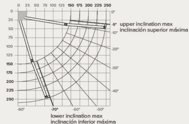
COMBI SINGLE-HOLE VERSION / VERSIÓN MONOAGUJERO
